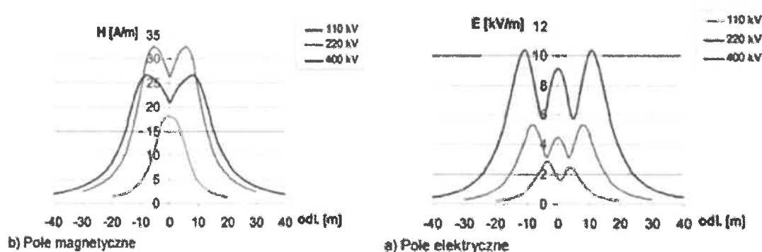
Rysunek 6 Natężenie PE i PM pod liniami WN
