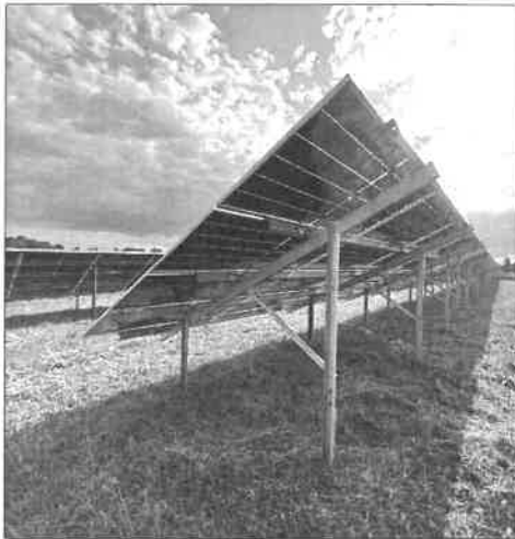
Zdjęcie 3 Konstrukcja wsporcza
