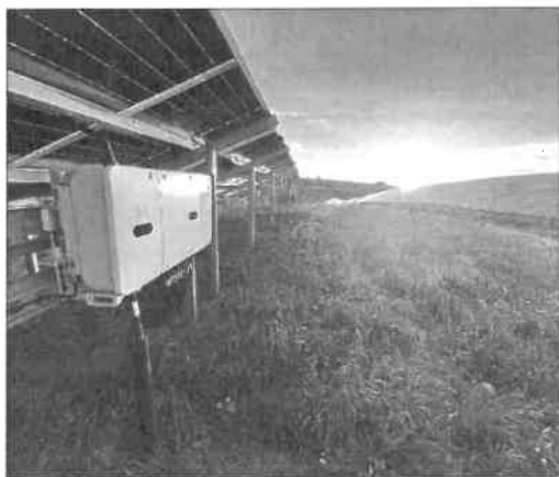
Zdjęcie 5 Inwerter – montaż na konstrukcji
