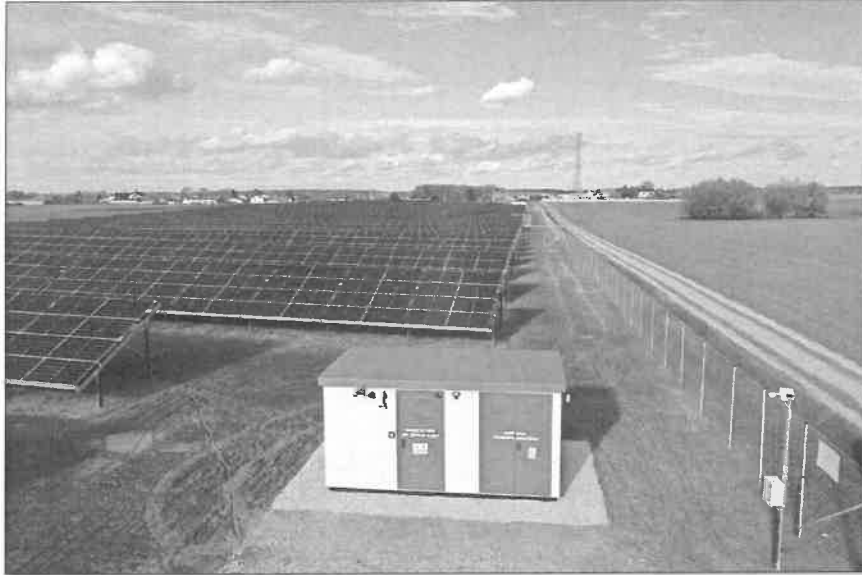
Zdjęcie 12 Plac pod stacją trafo.
