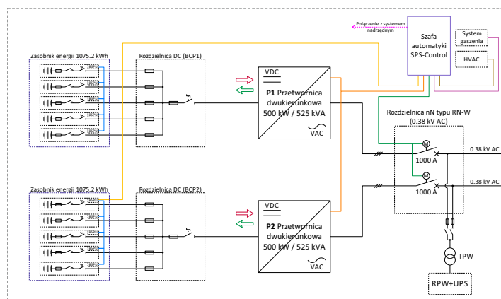
Schemat elektryczny
