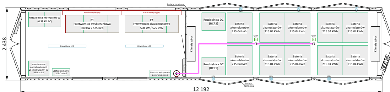
Widok z góry/rozmieszczenie aparatury
