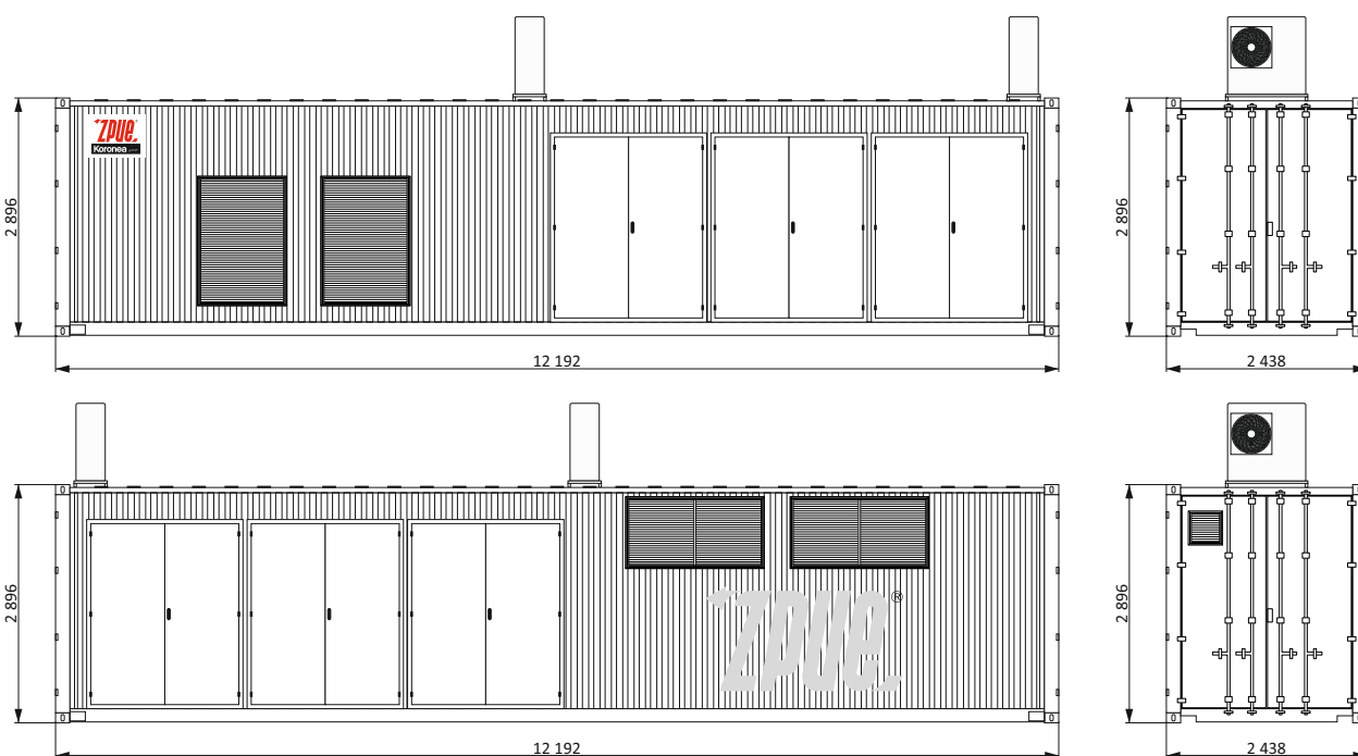
Elewacje
